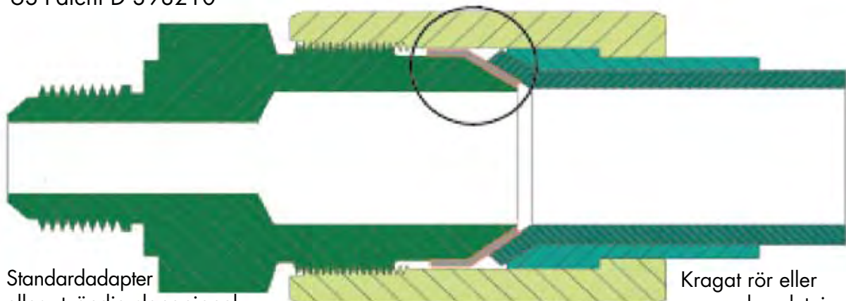
FLARETITE® TÄTNING US Patent D 398210
